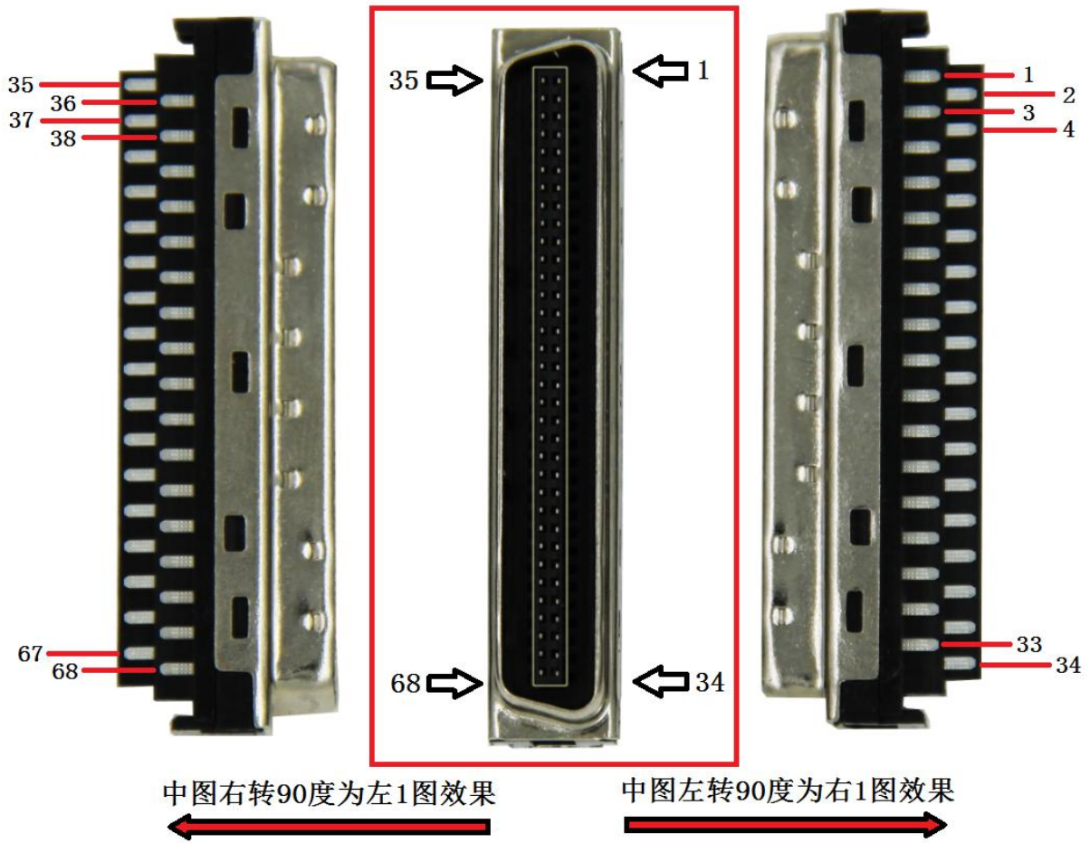
图 0-2 线缆焊接头标注
