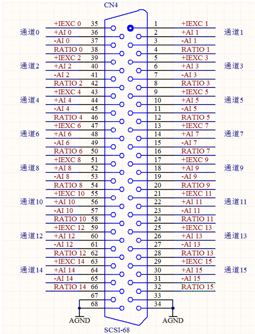
图 0-3 SCSI-68 母座原理图
