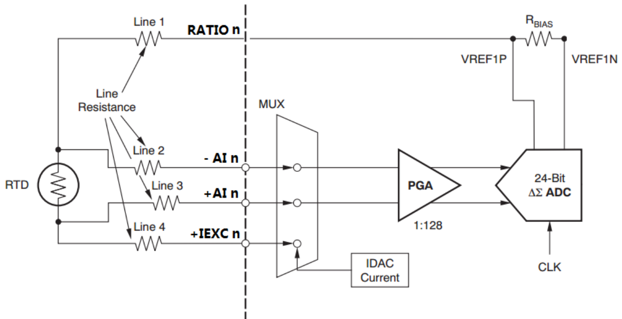
图 1-6 四线制接法
