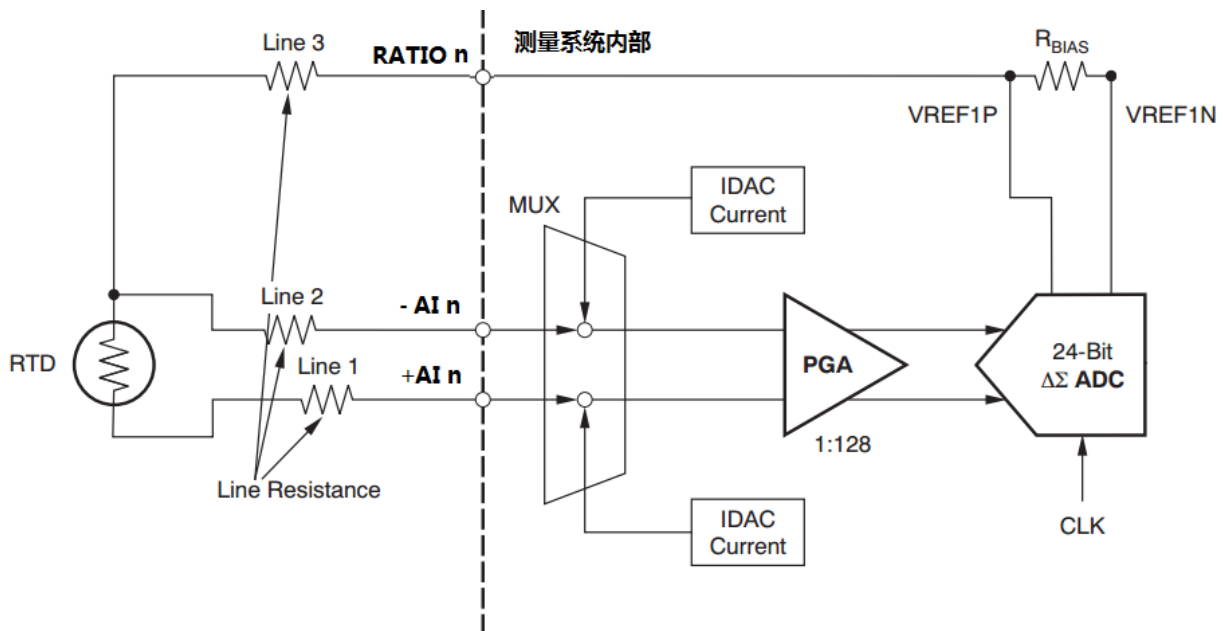
图 1-5 三线制接法
