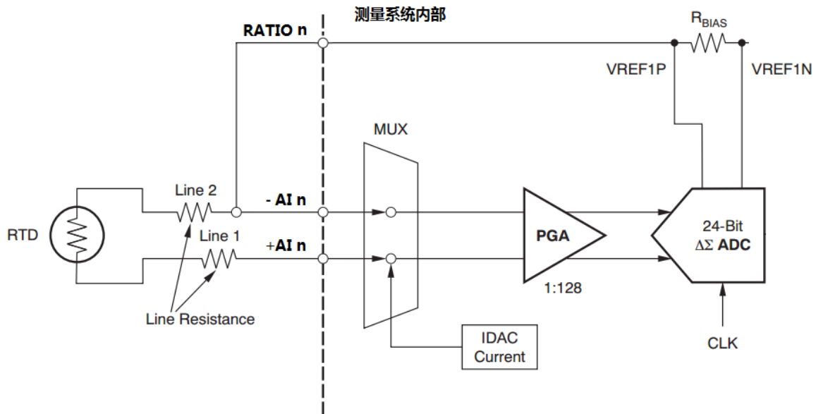
图 1-4 两线制接法
