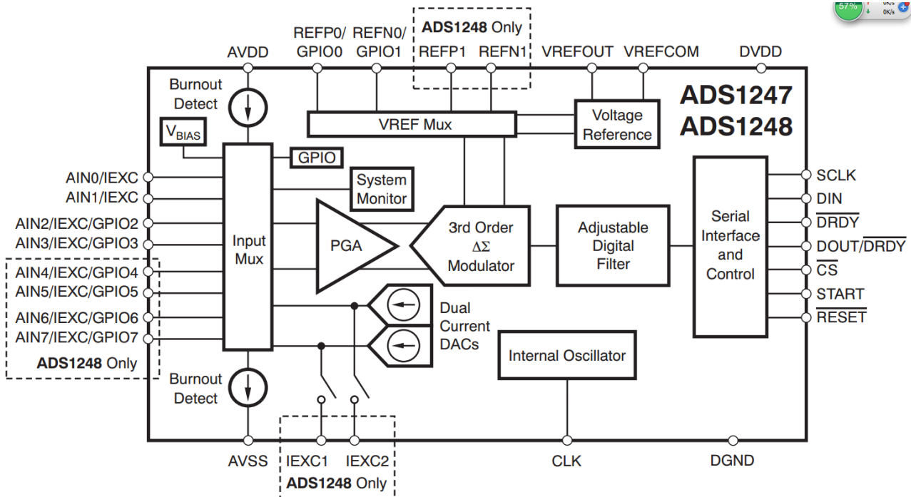
图 1-3 主测试芯片功能原理
