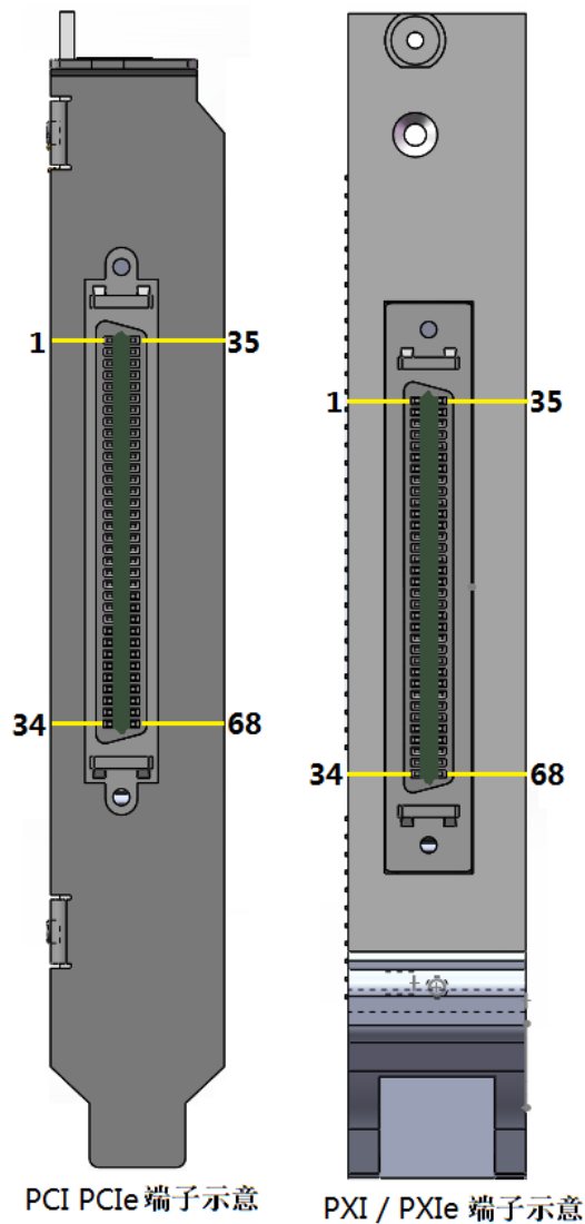
图 0-1 板卡接线端子示意图
