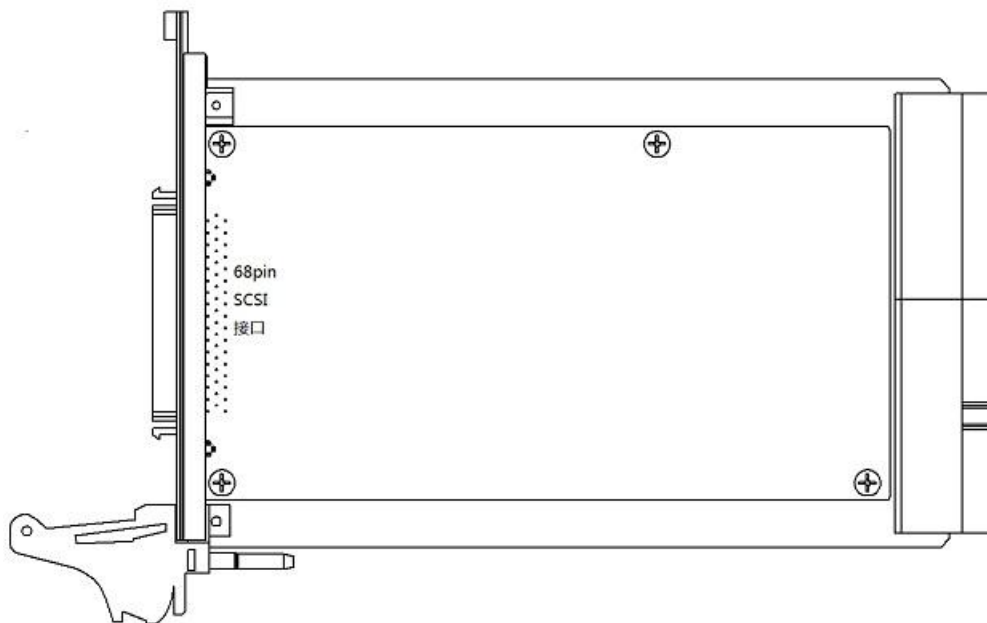
图 2-1 PXI-6183 产品布局图
