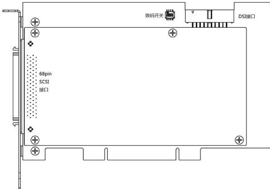
图 2-1 PCI-6261 产品布局图
