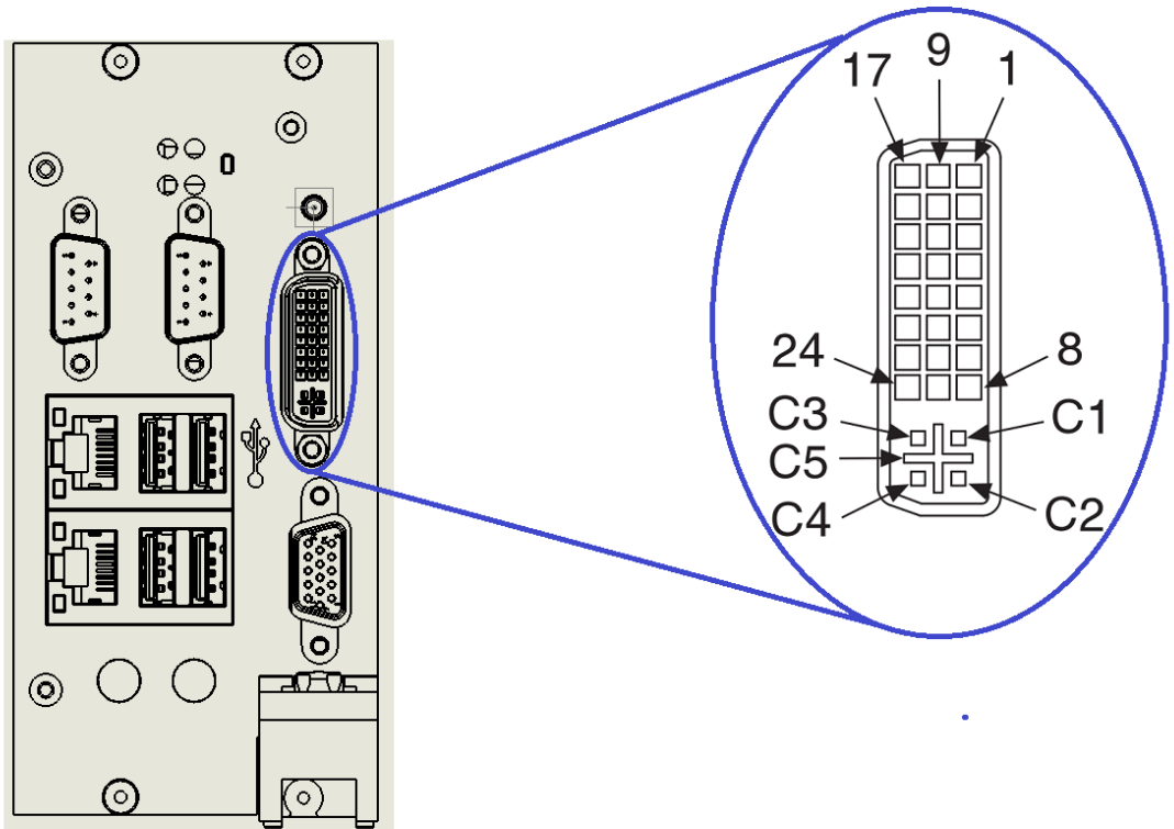
图 3-1 DVI 接口示意图
