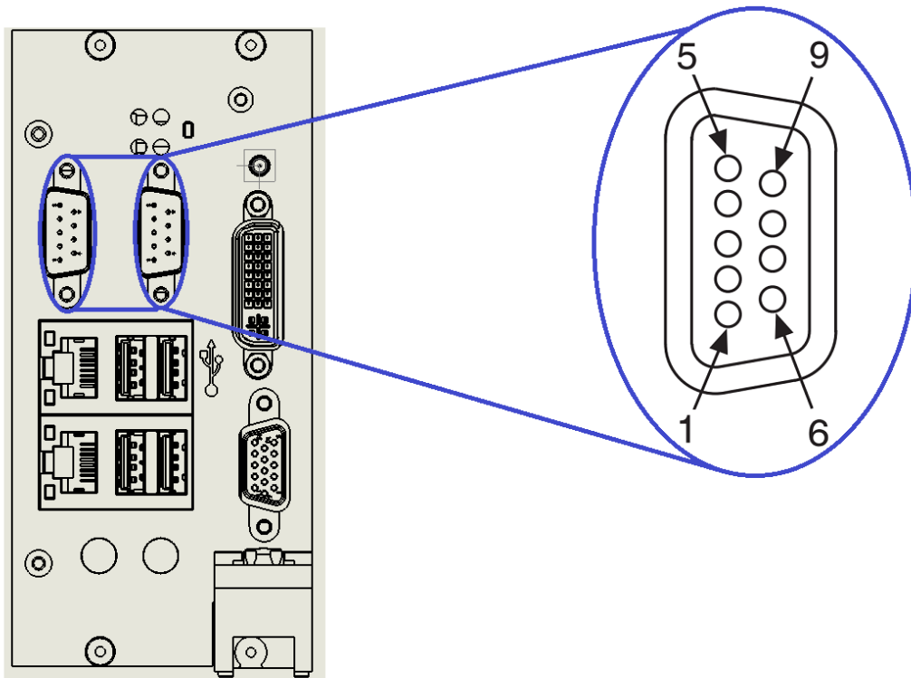
图 3-3 COM 接口示意图
