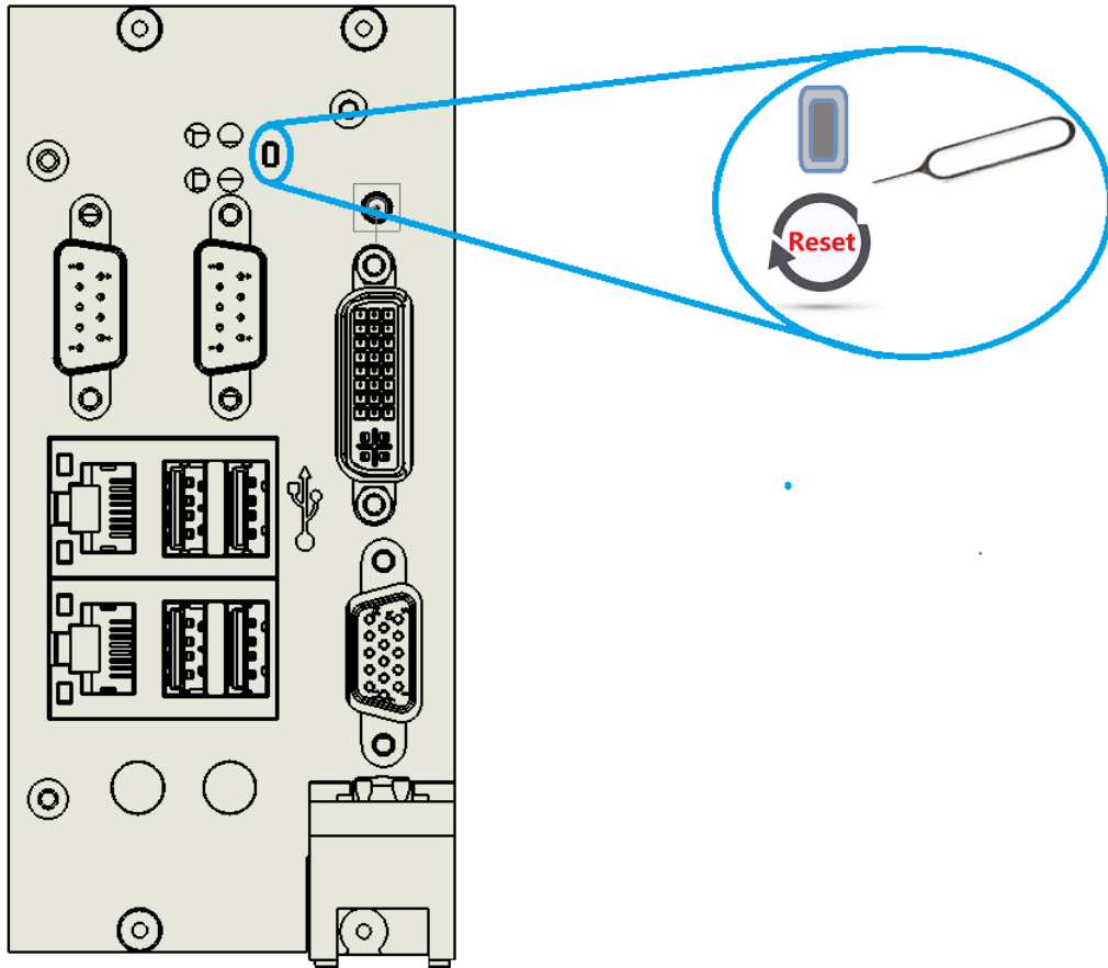
图 3-8 复位接口示意图
