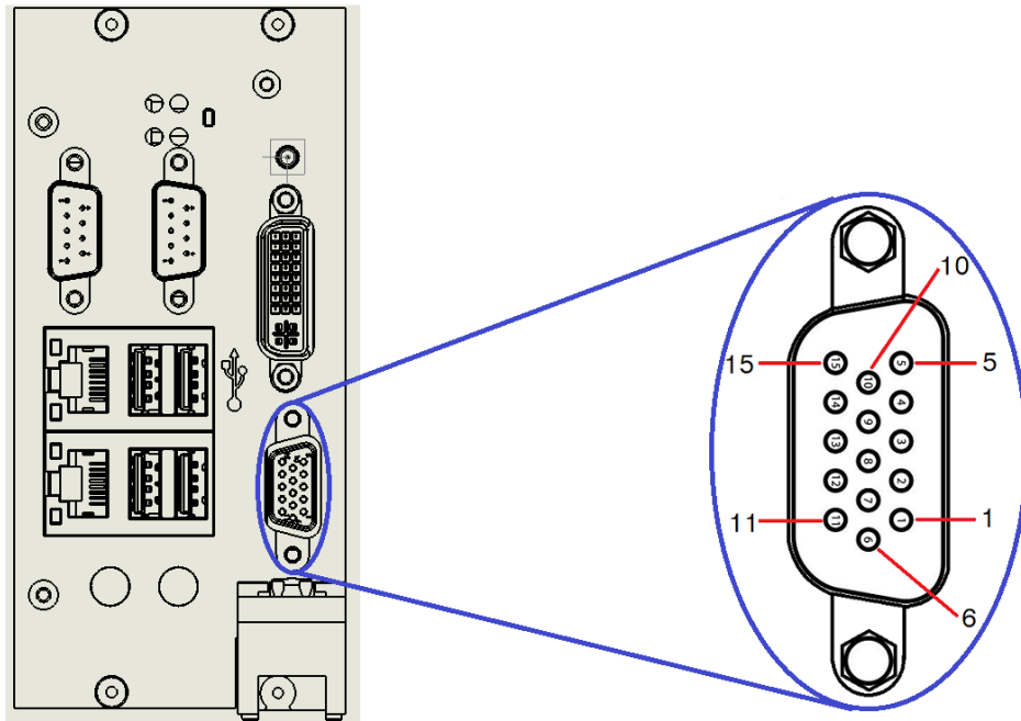
图 3-2 VGA 接口示意图
