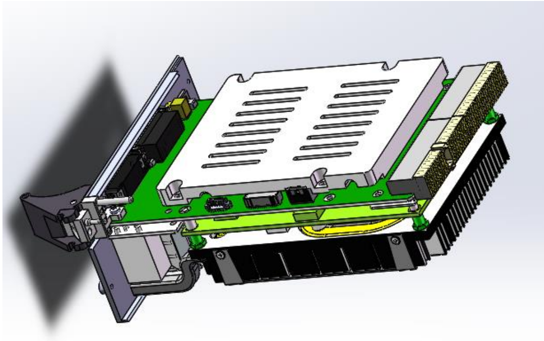
图 2-2 PXI-3871 产品侧视布局图 2
