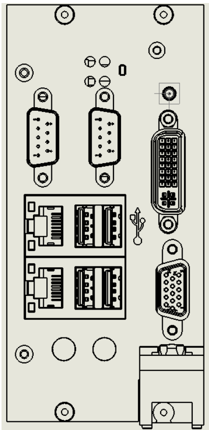
图 2-3 PXI-3871 产品面板布局图
