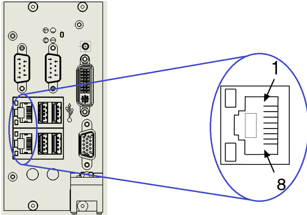
图 3-4 以太网接口示意图
