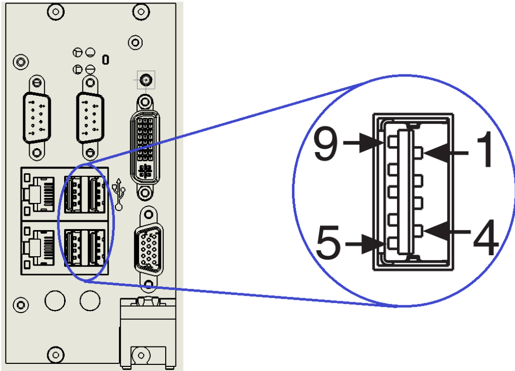
图 3-5 USB3.0 接口示意图
