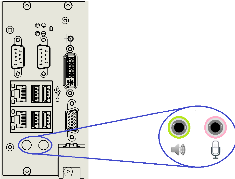
图 3-7 音频接口示意图
