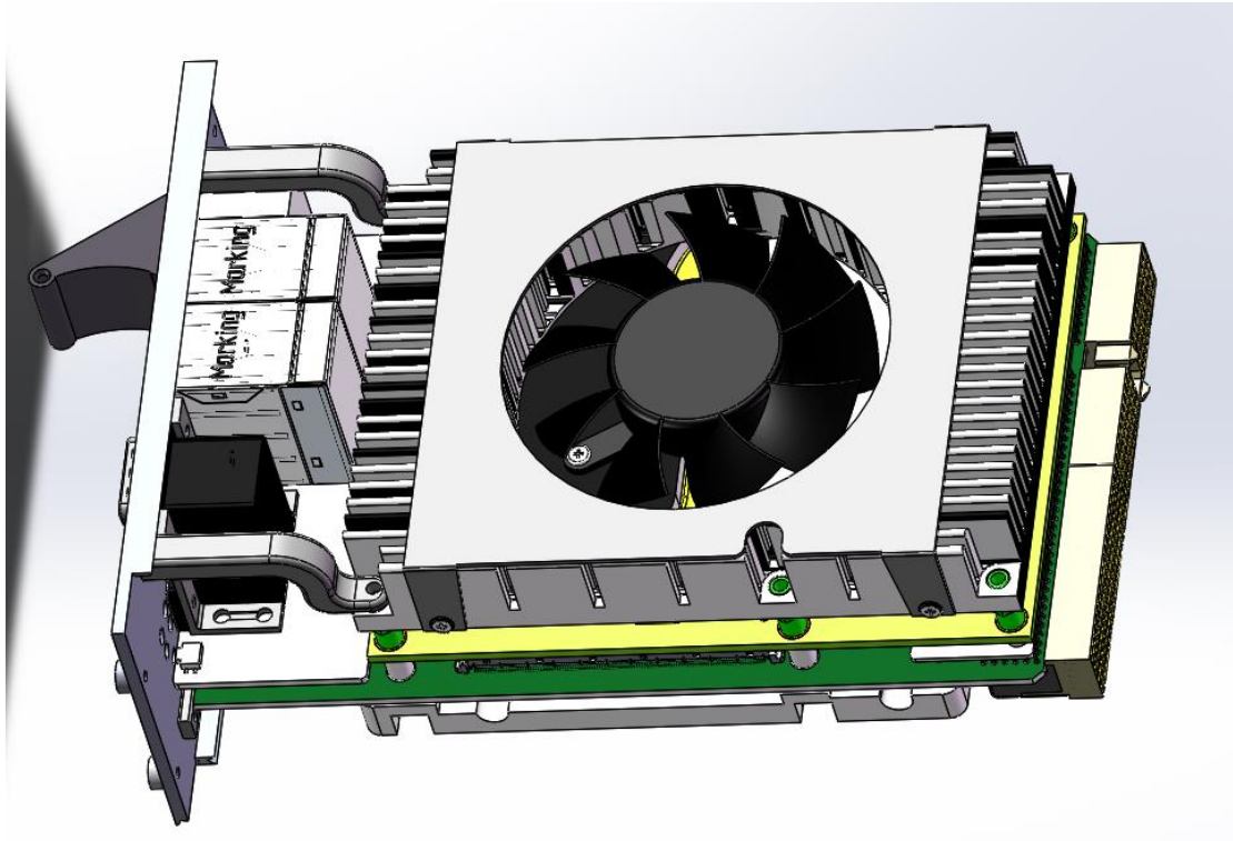
图 2-1 PXI-3871 产品测试布局图 1
