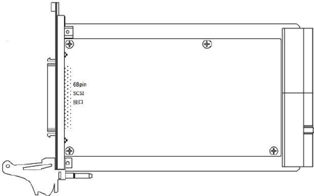
图 2-1 CPCI-7864 产品布局图
