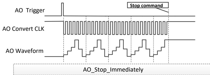
图 4-1 AO 停止模式 0
