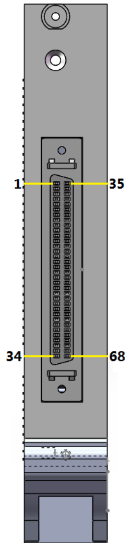
PXI 端子示意
