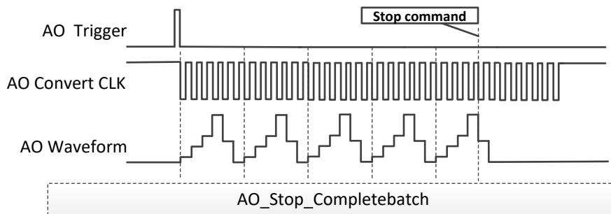
图 4-2 AO 停止模式 1
